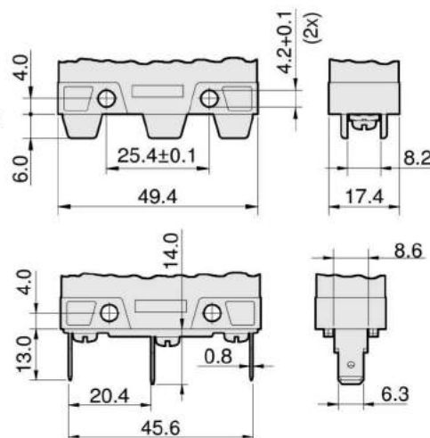
Terminal de Tornillo
