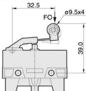
Actuador e Palanca con Rodillo
